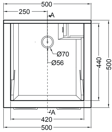
PIANTA
