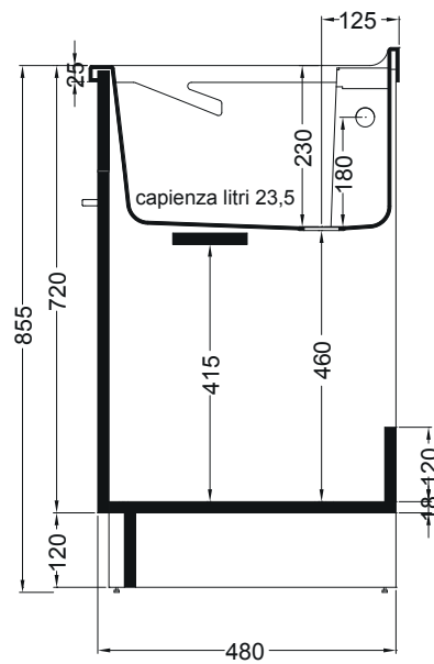
SEZIONE A-A'
